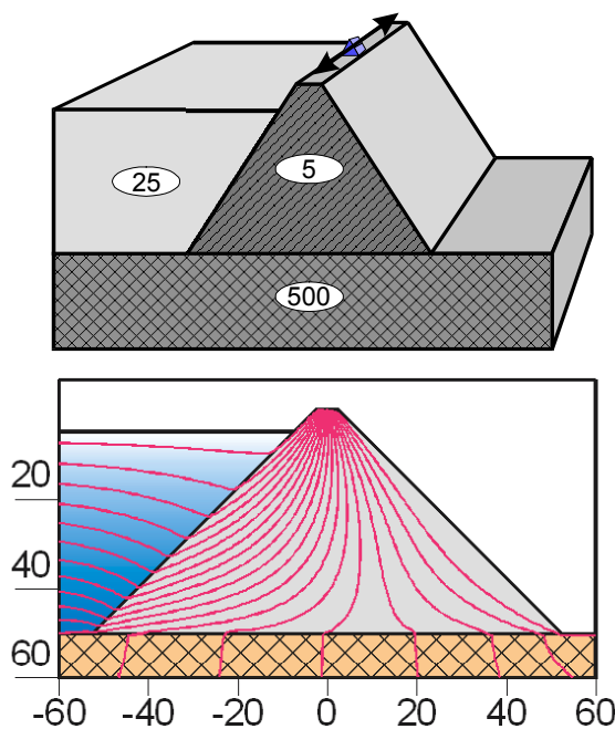
Рис. 3. Объемная модель земляной плотины.
