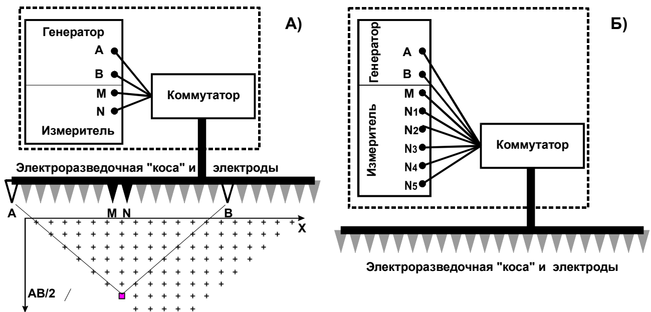
Рис. 1. Схемы многоэлектродной (А) и многоканальной (Б) аппаратуры.
