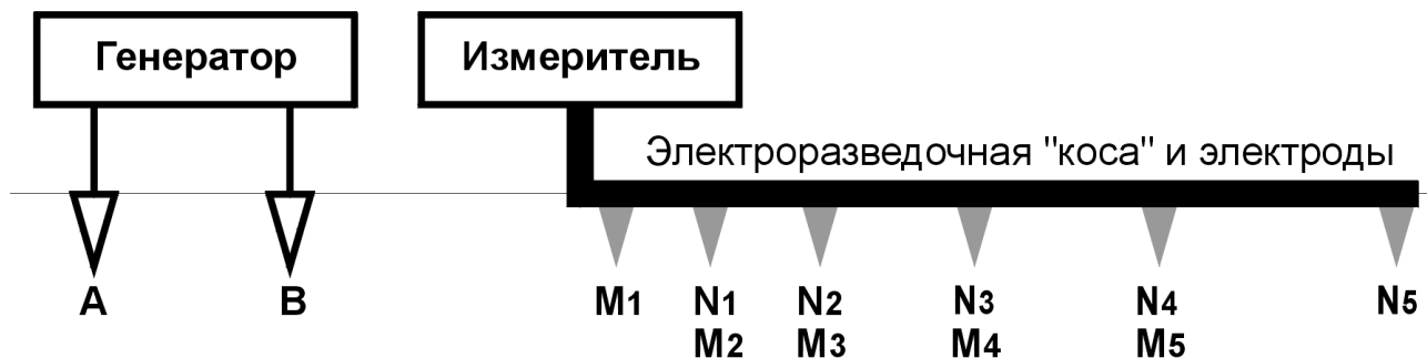
Рис. 1. Схема многоканальной аппаратуры.
